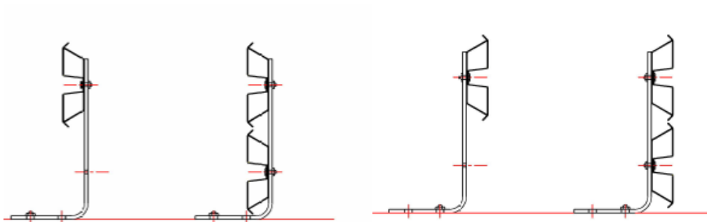
vangrail type B op verende bufferpaal
